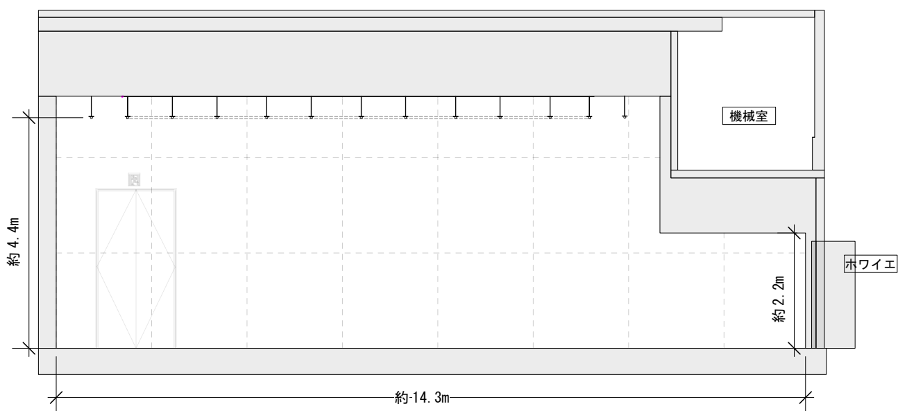
断面図 (1/100)
