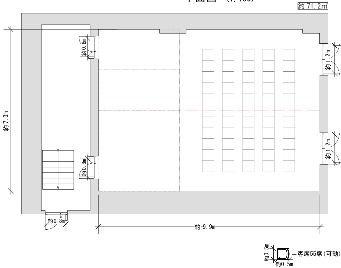
平面図 (1/100)
