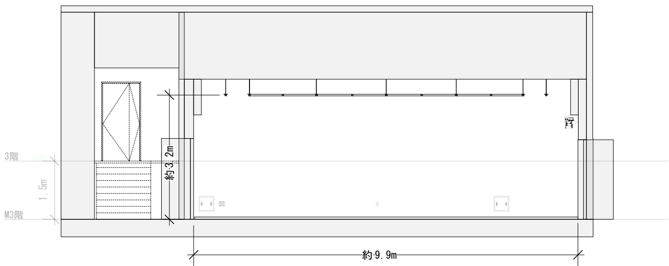
断面図 (1/100)
