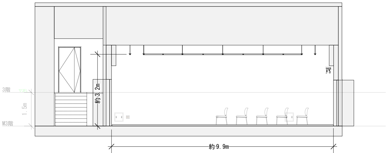
断面図 (1/100)
