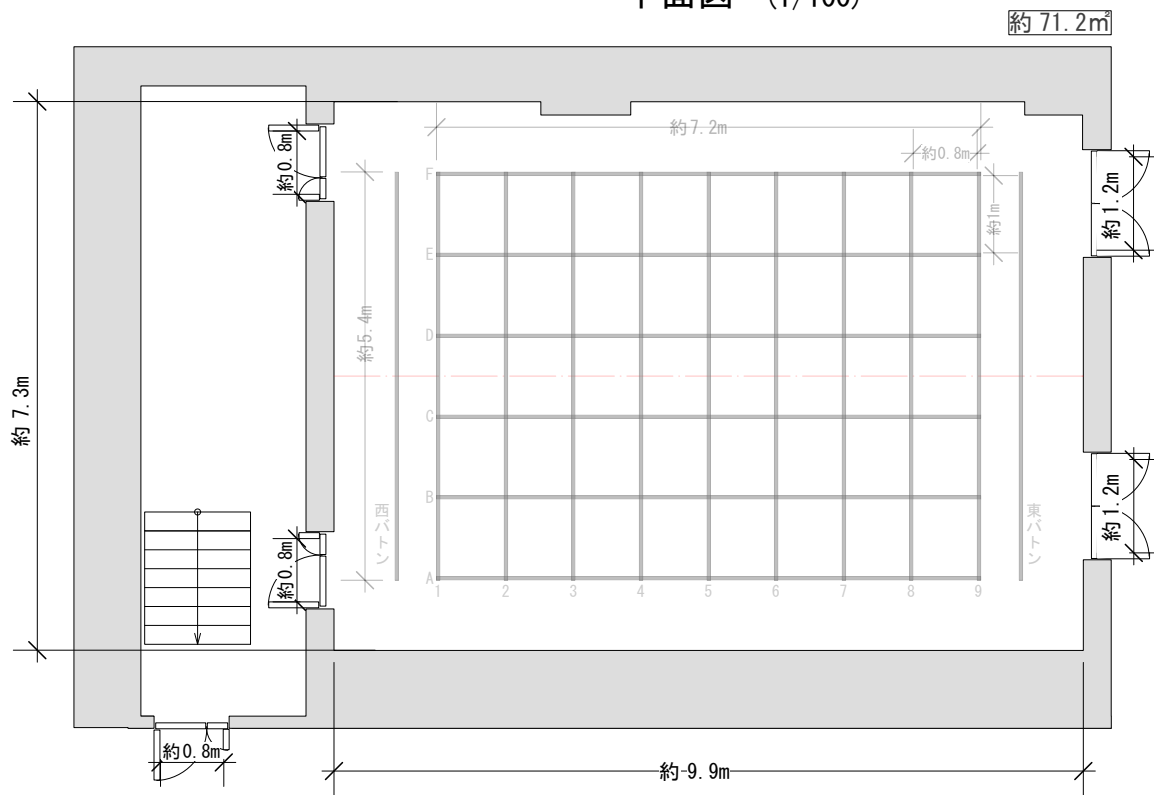
平面図 (1/100)
