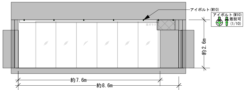
断面図 (1/100)
