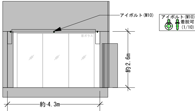
断面図 (1/100)
