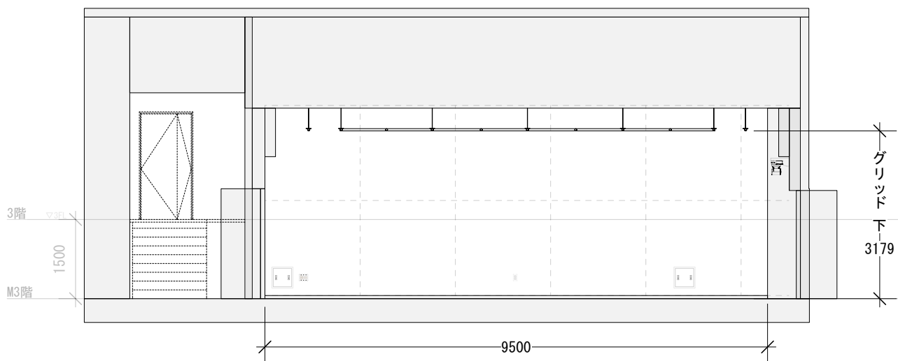
断面図 (1/100)
