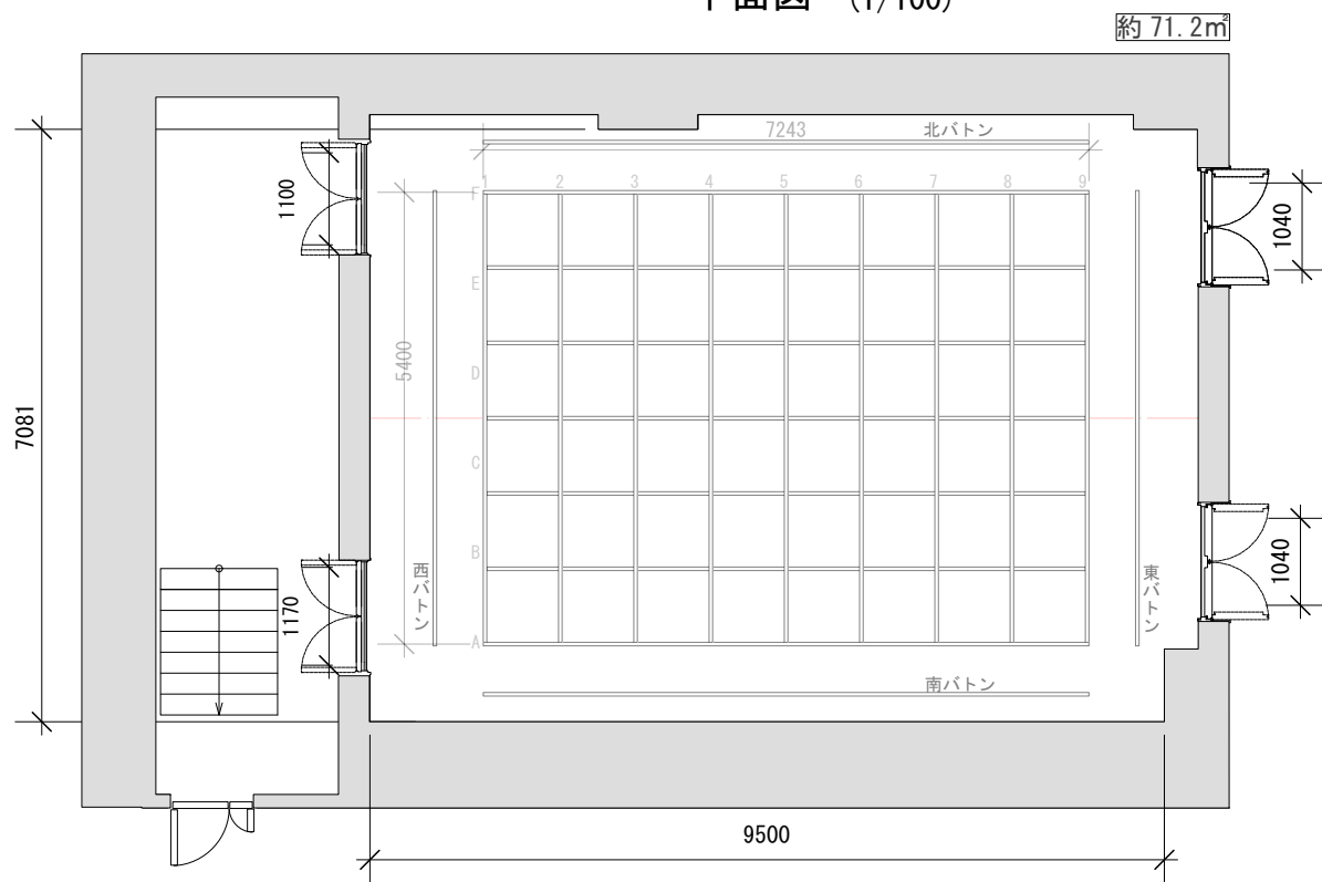
平面図 (1/100)
